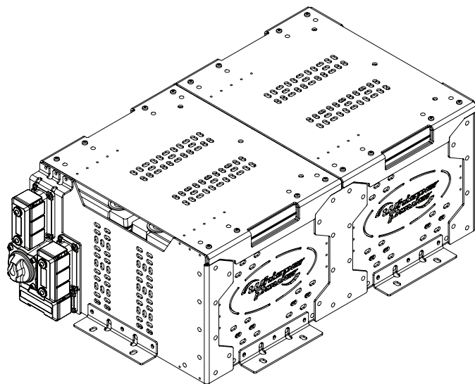
Battery Module
